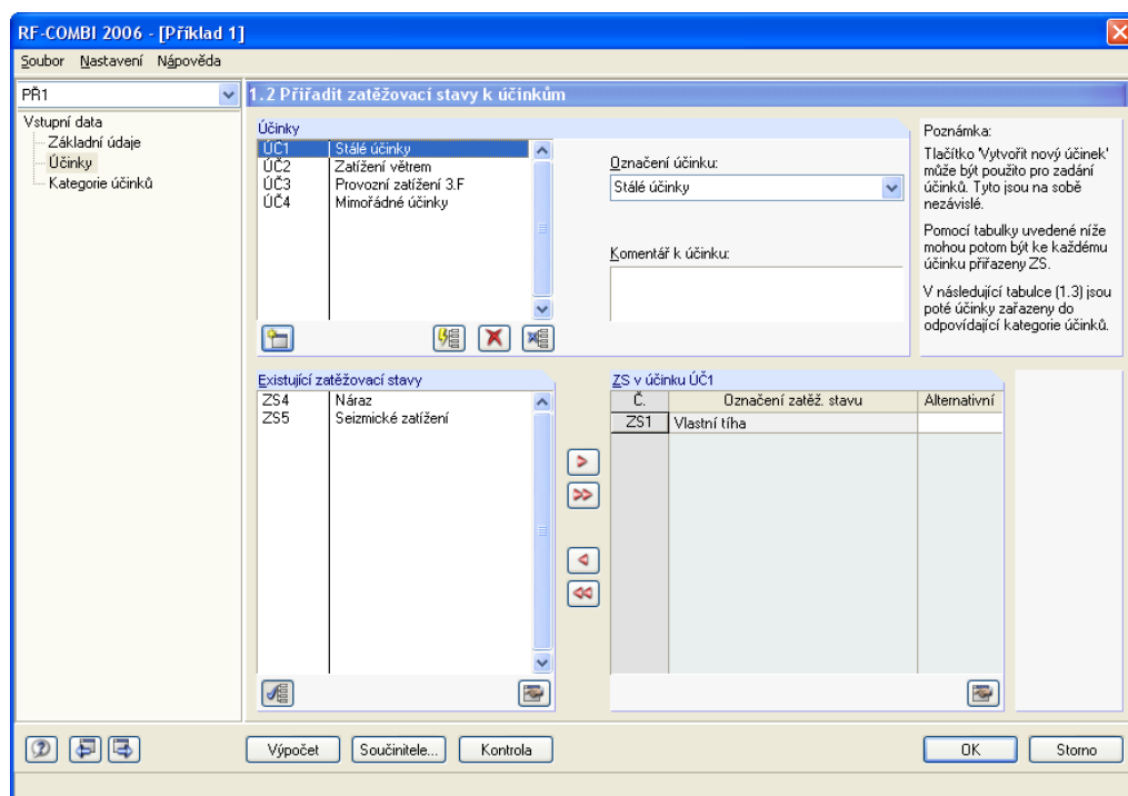
Obr. 3.22: Dialog 1.2 Účinky
