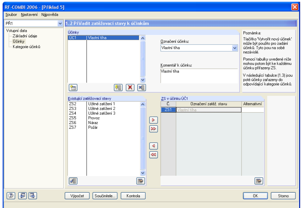
Obr. 5.27: Dialog 1.2 Účinky
