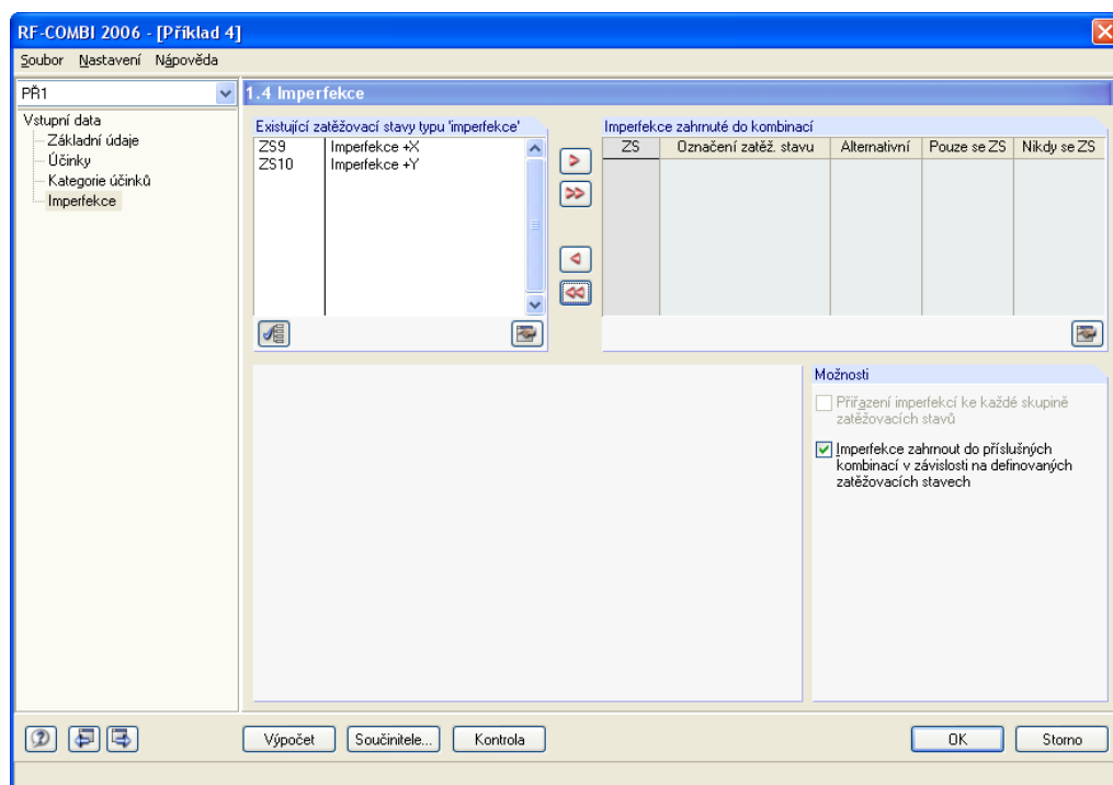
Obr. 3.18: Dialog 1.4 Imperfekce
