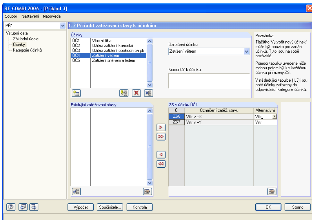
Obr. 5.14: Dialog 1.2 Účinky
